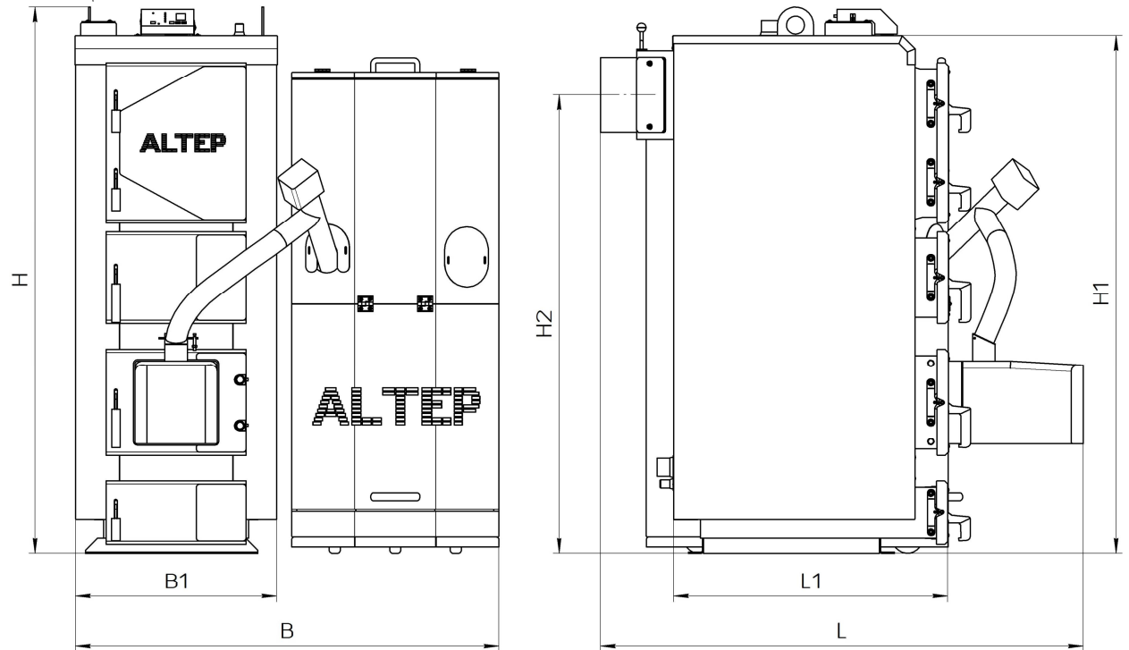
Рисунок 1 – Габаритне креслення котла типу KT-2E-PG
